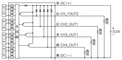
PF2W201 PNP (4出力)
