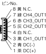
電源・出力接続ケーブル (付属品)
