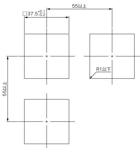
パネルカット寸法
