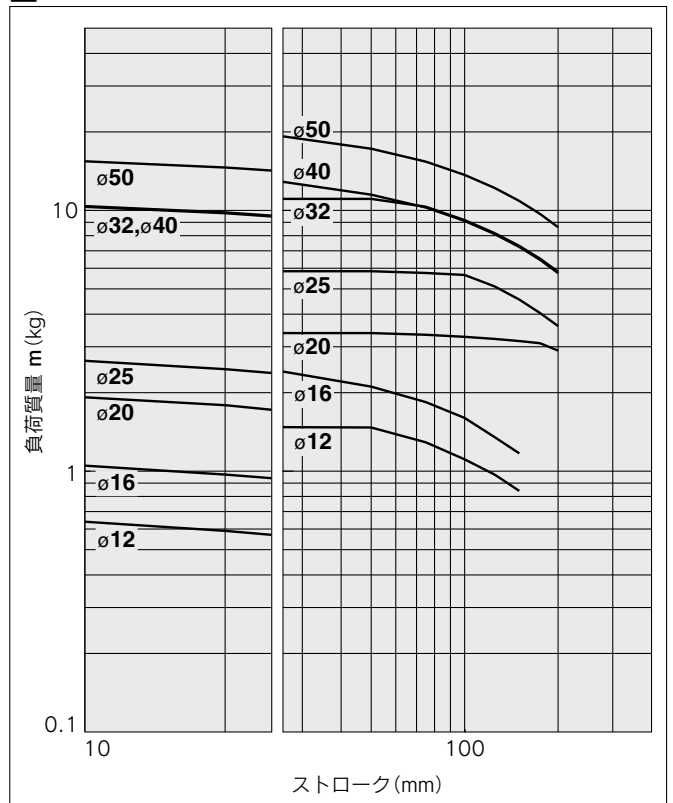
8 L=100mm V=400mm/s
