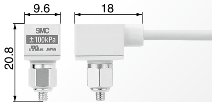
For PSE54□-M3
