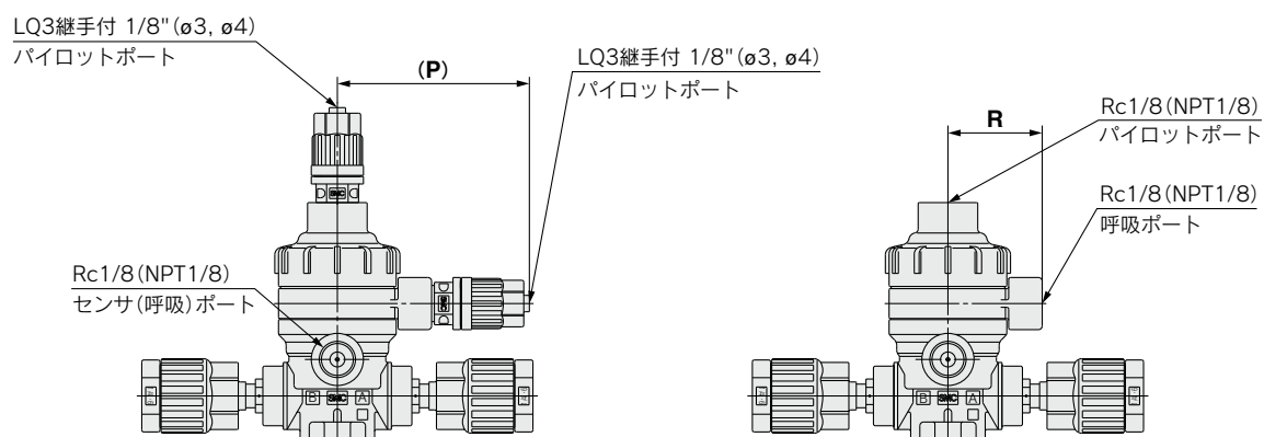
LVQ \square_{\frac{1}{2}} S-Z \square 寸法表(N.O.弁, 複動弁)
